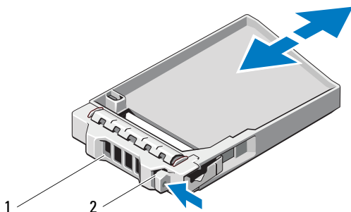
图 16-3. 卸下和安装 2.5 英寸硬盘驱动器挡片（仅限 MD3620f）
